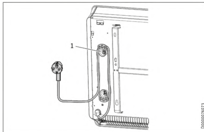
1 Support du câble d'alimentation
